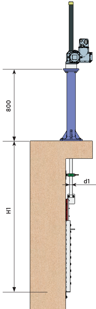
STANDARD-FLURSÄULE
