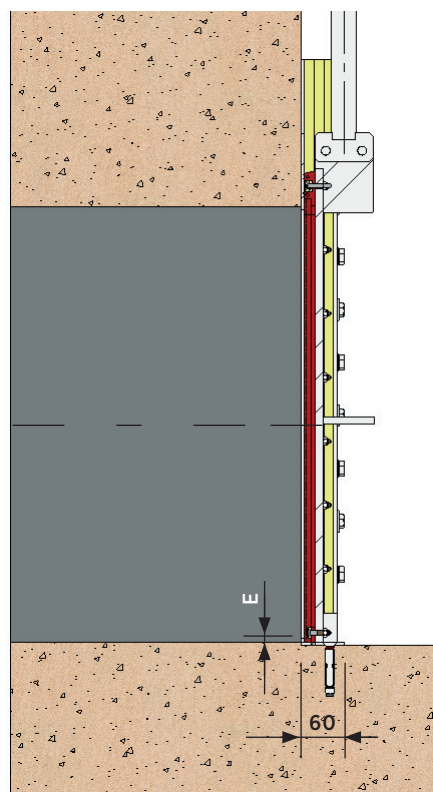
SEITENANSICHT
