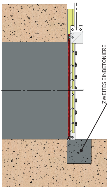
SEITENANSICHT
