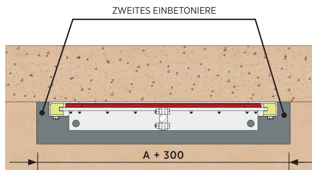
DRAUFSICHT
