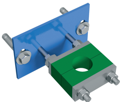
SPINDELHALTER
