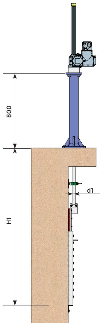
STANDARD-FLURSAULE
