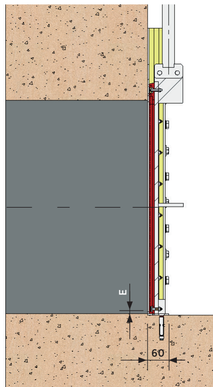
SEITENANSICHT
