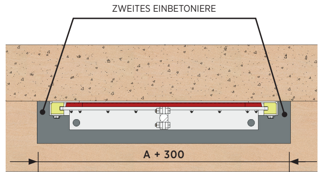
DRAUFSICHT
