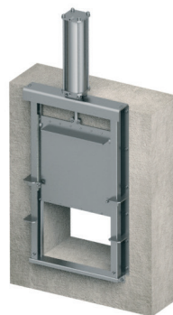
Fig. 13 ACCIONAMENTO NEUMÁTICO
