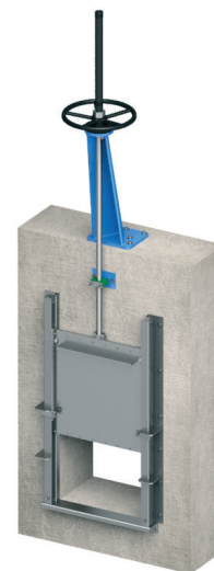
Fig. 14 VOLANTE FUSO ASCENDENTE
