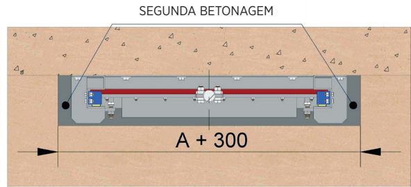
VISTA EM PLANTA
